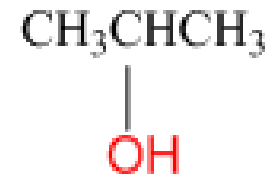
2-пропанол
