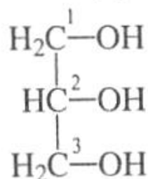
1,2,3-пропантриол (глицерол)
