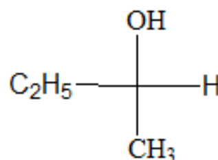
L-бутанол-2
