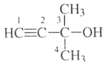
3-метил-1-бутин-3-ол (3-метил-3-хидоксибутин)
