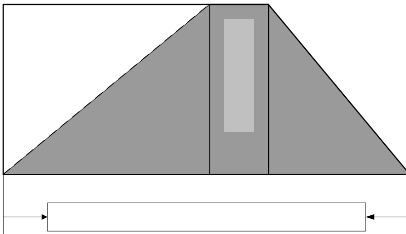
Фиг. 5 Теоретичен модел на Шефийлд
